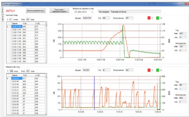
▲ Удаленный просмотр аварийных записей
