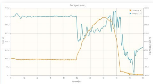
▲ График быстрого следа в WEB интерфейсе
