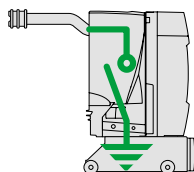
Устройство заземления сборных шин на выкатной тележке
