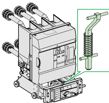
Механизм блокировки двери отсека выключателя
